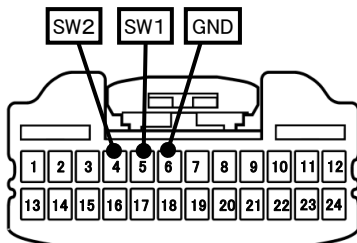
24Pコネクタ(白)
