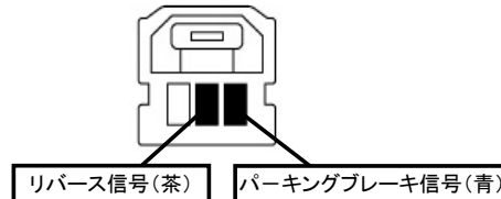
変換ハーネス側のコネクタ3P(灰)
